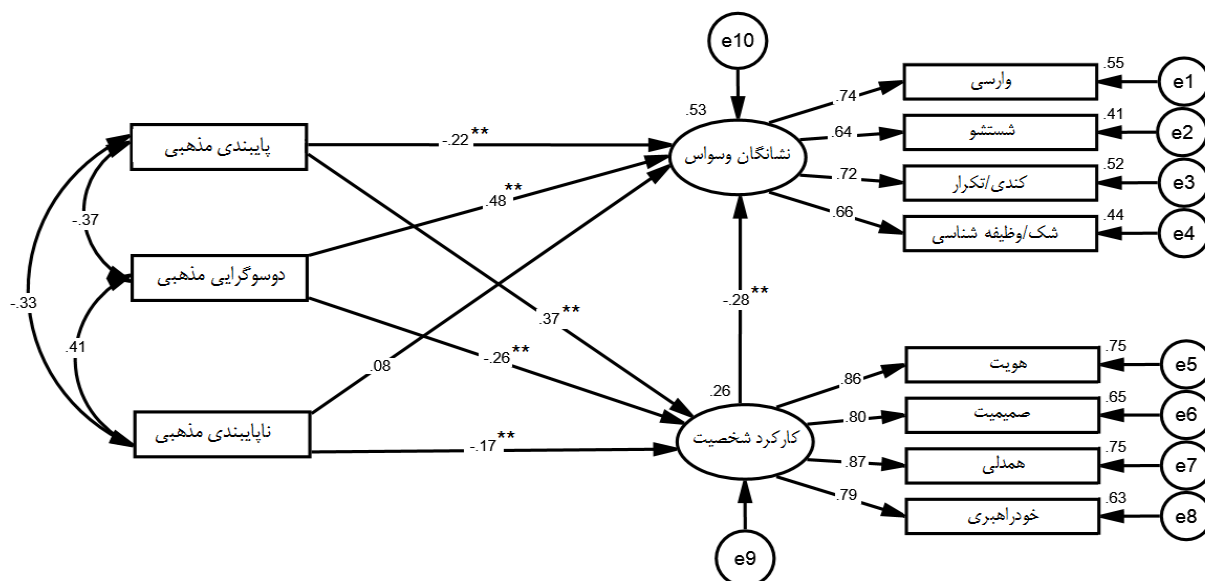
شکل ۱ مدل ساختاری پژوهش مربوط به پژوهش
